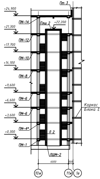
Разрез 5-5
