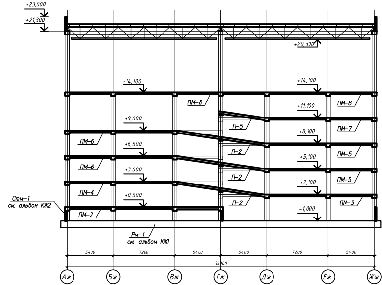
Разрез 3-3
