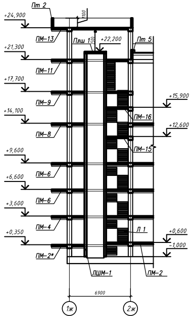
Разрез 4-4
